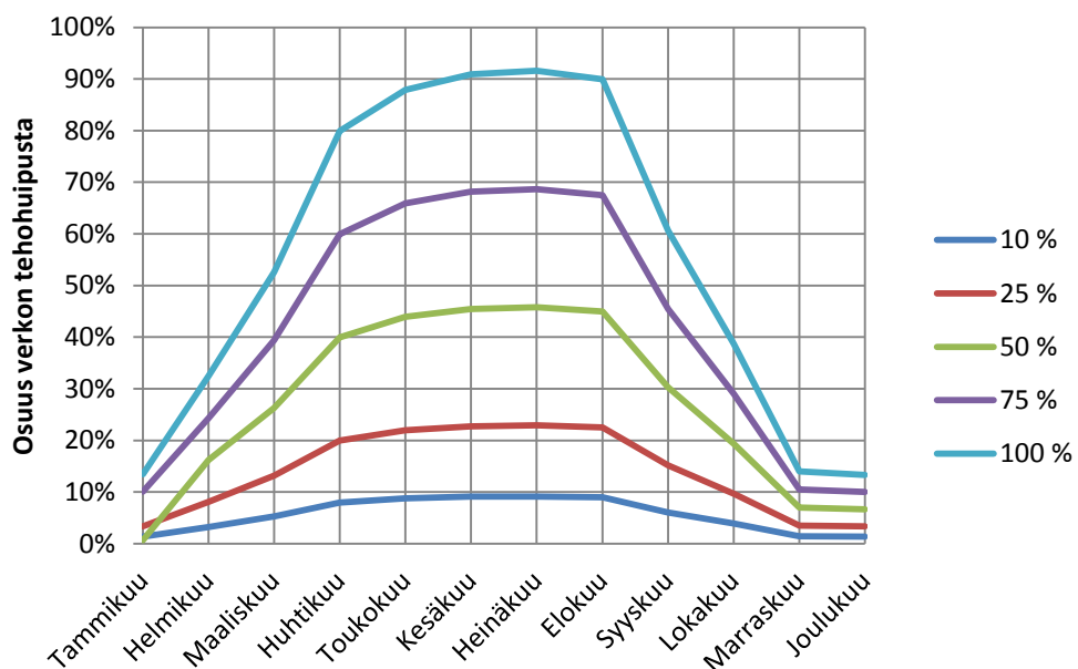
Kuva 6.1. Aurinkosähkön potentiaalin eri käyttöasteilla tuotetun huipputehon osuus Tampereen sähkön siirron huipputehosta klo 11 - 15 välisenä aikana.
