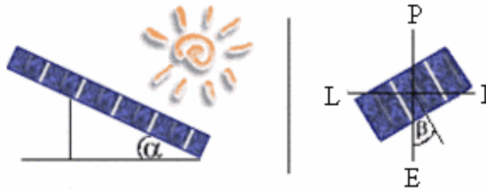
Kuva 2.1. Paneelin kallistuskulma \alpha sekä suuntakulma \beta [10].
