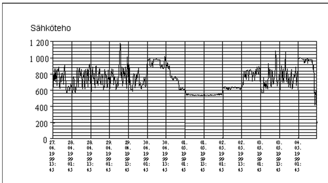
Kuva 3. Paineilmajärjestelmän sähkökuormituksen (15 min keskiteho) vaihtelu mittausajankohtana.
