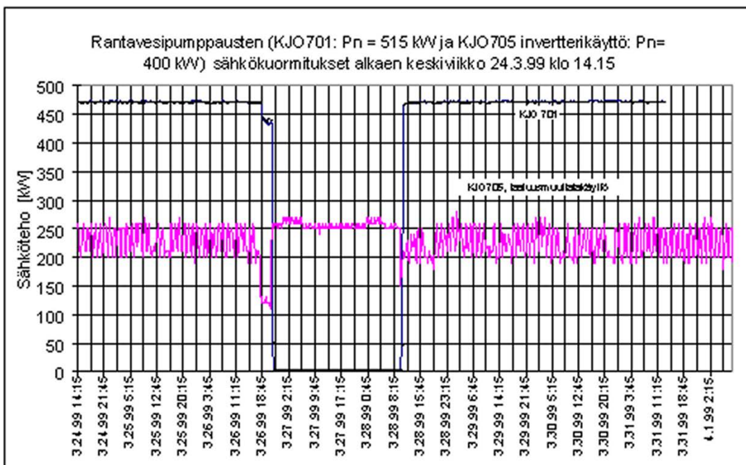
Kuva 4. Rantavesipumppujen sähkökuormituksen (15 min keskiteho) vaihtelu mittausajankohtana.
