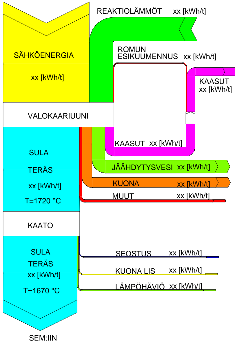
Kuva 1. Esimerkki osaprosessin taseesta.
