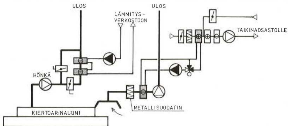
Kuva 44. Lämpimien tuotteiden lämmön hyödyntäminen esimerkiksi palamisilman esilämmitykseen.
