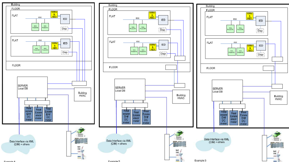
Kuva 1. Liittyä kohtaan 2: eräitä esimerkkejä kiinteistön mittaus- ja ohjausjärjestelystä.
