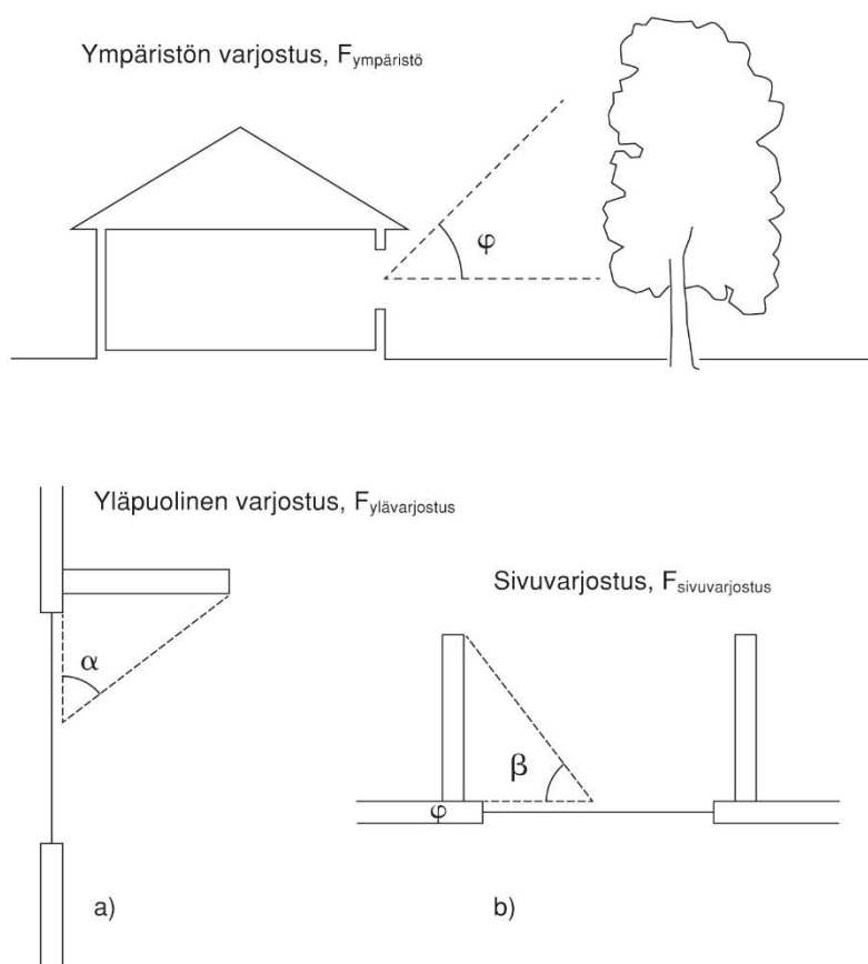
Kuva 5.1. Varjostuskulmien määritelmät.
