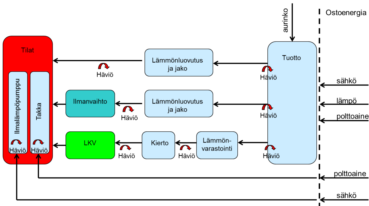
Kuva 6.1. Lämmitysjärjestelmälaskennan periaate.
