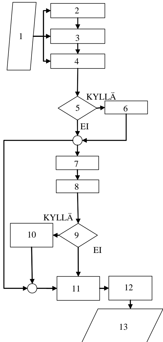
Kuva 2. Laskentajärjestyksen vuokaavio
