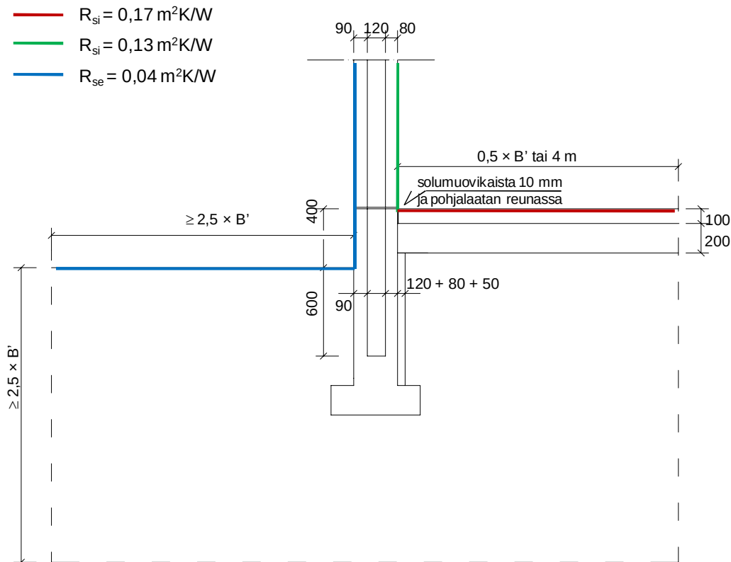
Kuva 42. Kuvan 41 detaljista yksinkertaistettu malli ja pintavastusten arvot. Perustapauksessa laatan reunan solumuovikaistan leveys oli d = 10 mm.
