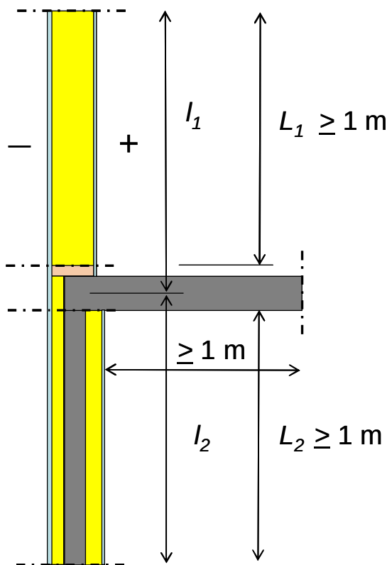
Kuva 2. Esimerkki alemman ja ylemmän kerroksen seinien ja välipohjan liitoksen kylmäsillasta. Tarkastelugeometria rajataan pistekatkoviivojen kohdalta. Kuvan periaate on lähteestä Gustavsen et al. 2008.
