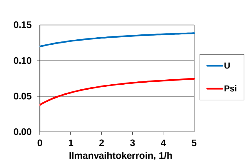
Kuva 64. Ryömintätilan ilmanvaihtokertoimen (vaihtoa tunnissa) vaikutus alapohjan lämmönläpäisykertoimeen U ja liitoksen viivamaiseen lisäkonduktanssiin \Psi .
