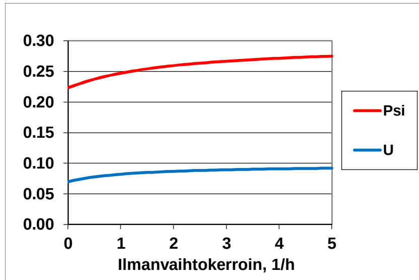
Kuva 46. Ryömintätilan ilmanvaihtokertoimen (vaihtoa tunnissa) vaikutus alapohjan lämmönläpäisykertoimeen U ja liitoksen viivamaiseen lisäkonduktanssiin \Psi .
