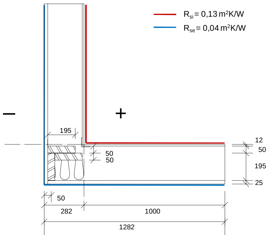
Kuva 21. Kuvan 20 detaljista yksinkertaistettu laskentamalli ja mallin pintavastukset.
