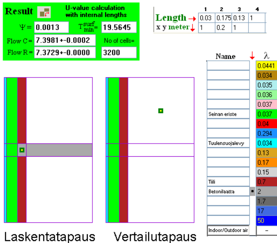
Kuva 70. Laskentamalli ja sen vertailutapaus tiiliseinän ja betonivälipohjan liitoksesta. Seinän eristepaksuus on 120 mm. Mitat vaaka- ja pystysuuntaan sekä materiaalien lämmönjohtavuudet käyvät ilmi kuvasta.
