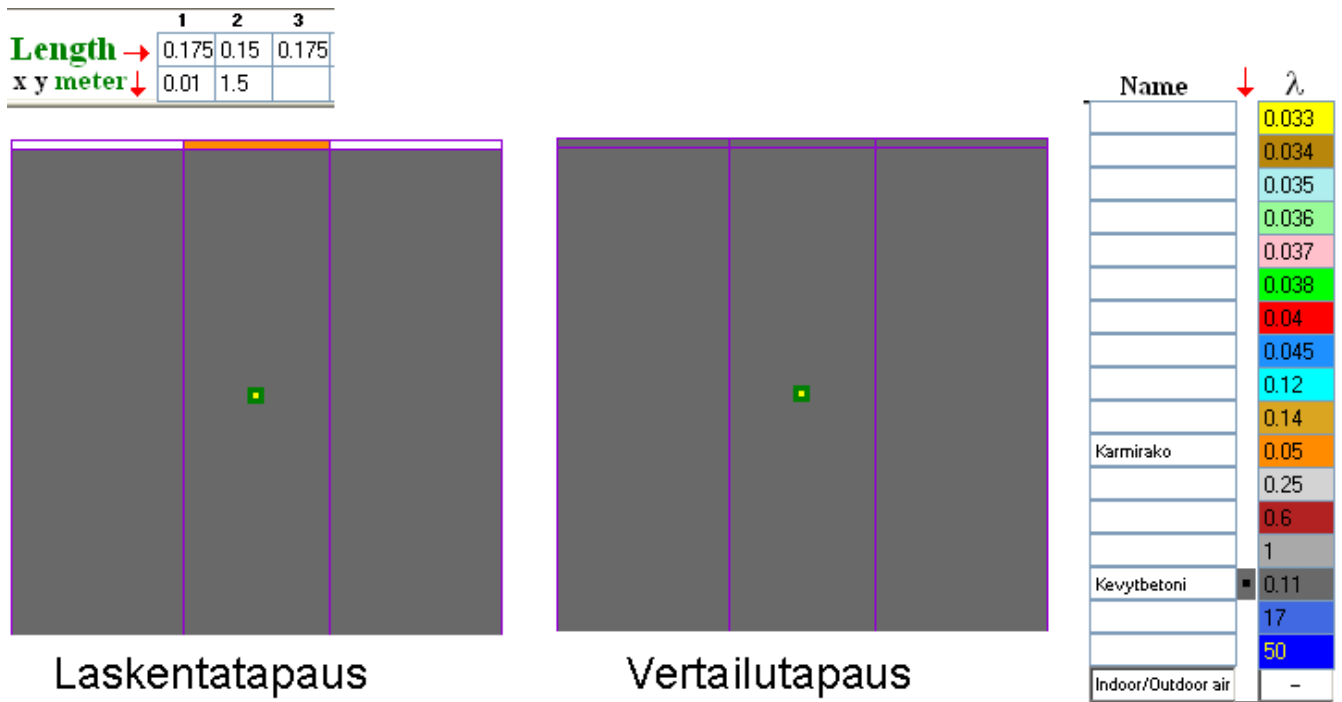
Kuva 82. Laskentamalli ja sen vertailutapaus ikkunan liitoksesta massiiviseen kevytbetoniseinään. Mitat vaaka- ja pystysuuntaan sekä materiaalien lämmönjohtavuudet käyvät ilmi kuvasta.
