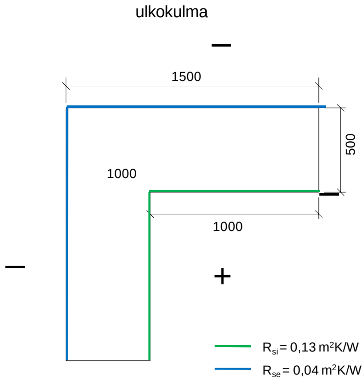
Kuva 76. Massiivisen kevytbetoniseinän ( d = 500 mm) ulkokulma.
