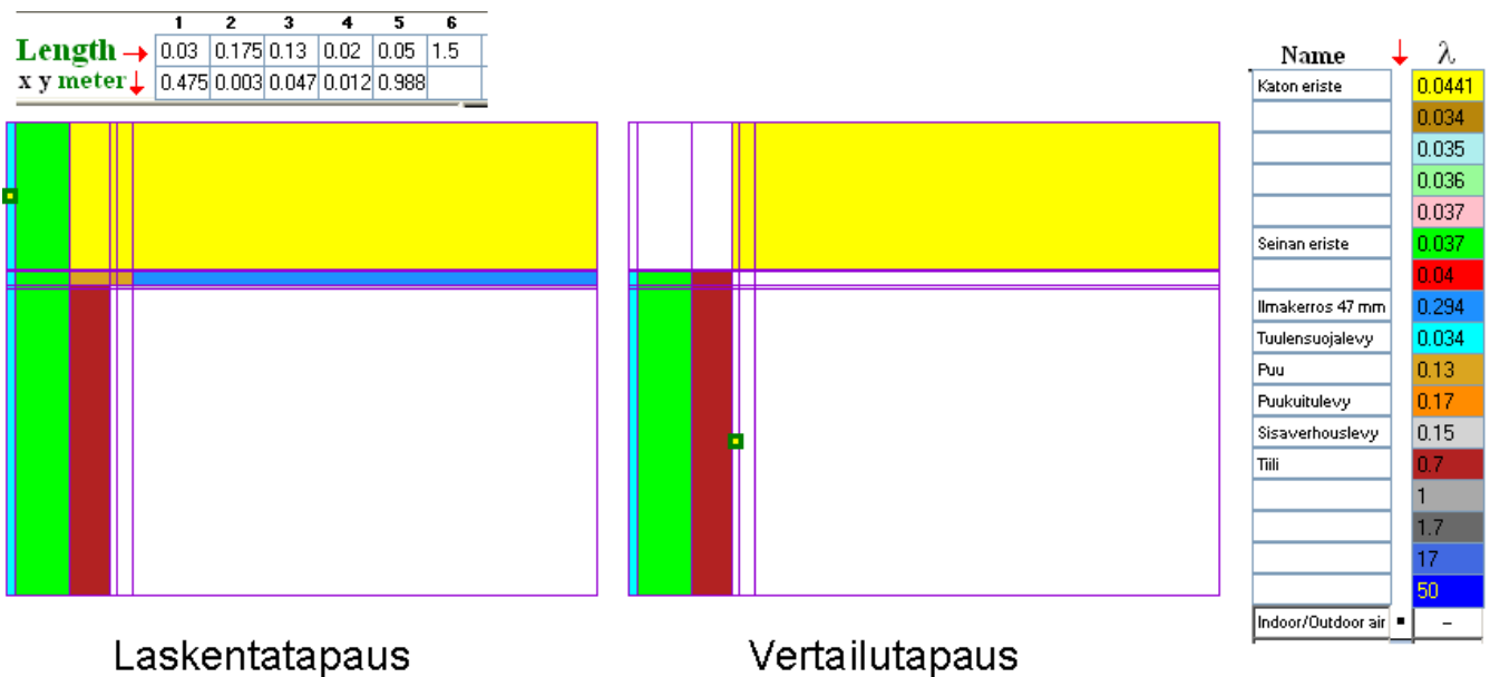
Kuva 67. Laskentamalli ja sen vertailutapaus tiiliseinän ja yläpohjan liitoksesta. Mitat vaaka- ja pystysuuntaan sekä materiaalien lämmönjohtavuudet käyvät ilmi kuvasta. Huomaa, että vertailutapauksen seinä ulottuu katon ilmaraon yläpinnan tasolle.
