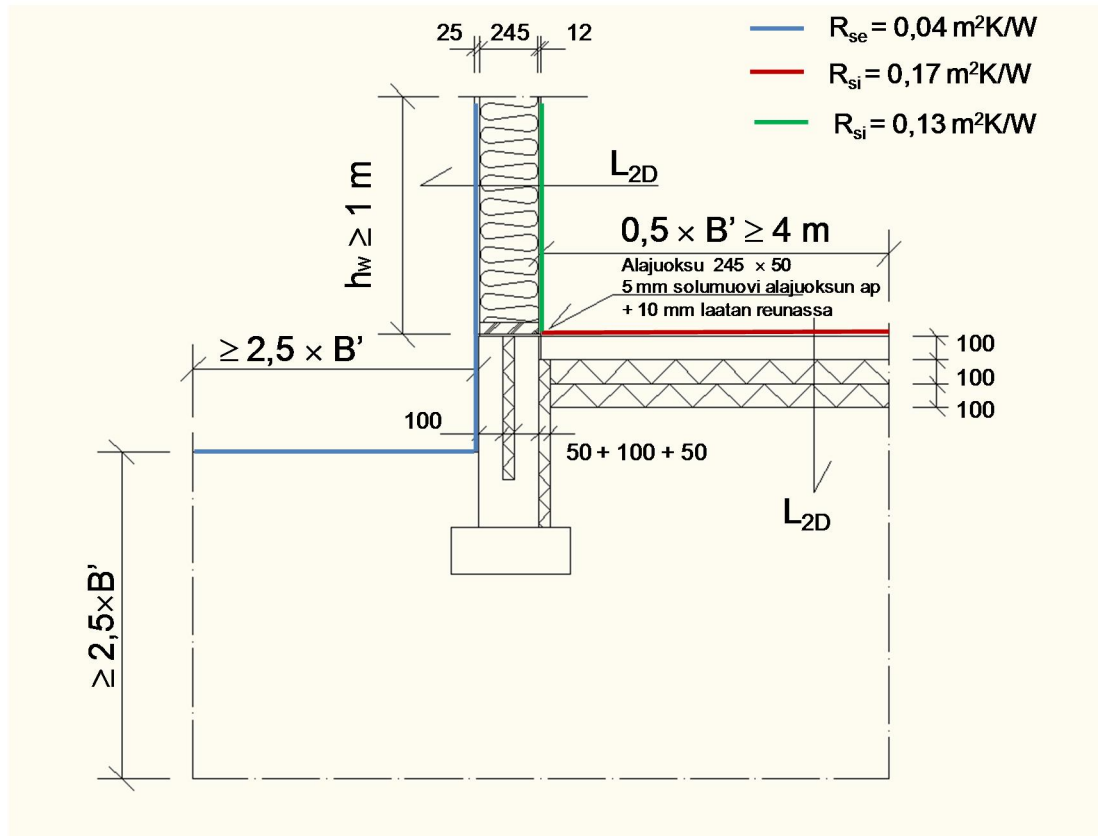
Kuva 14. Liitosdetaljin yksinkertaistettu malli ja päämitat.
