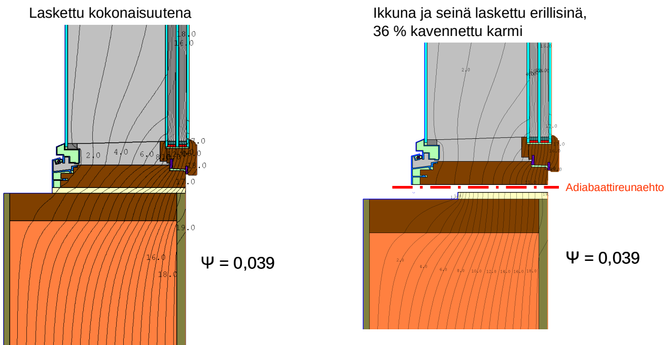
Kuva 34. Ikkunan MS3E laskennallinen karmisyvyys on 36 % todellista karmisyvyyttä pienempi kun käytetään adiabaattireunaehtoa.
