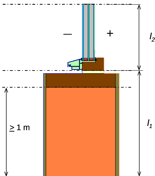
Kuva 31. Kiinteän kolmilasisen puu-alumiini-ikkunan kiinnitys puurankaseinään.
