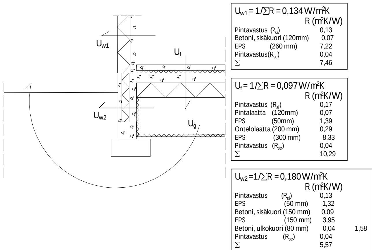
Kuva 45. Ryömintätillaisen alapohjan, eristetyn kiviseinän ja eristetyn pintalaatan liitos. Alapohjan ja ulkoseinän lämmönläpäisykertoimet U_{w1} = 0,134 \text{ W/m}^2\text{K} ja U_f = 0,097 \text{ W/m}^2\text{K} vastaavat ns. passiivitalon arvoja.
