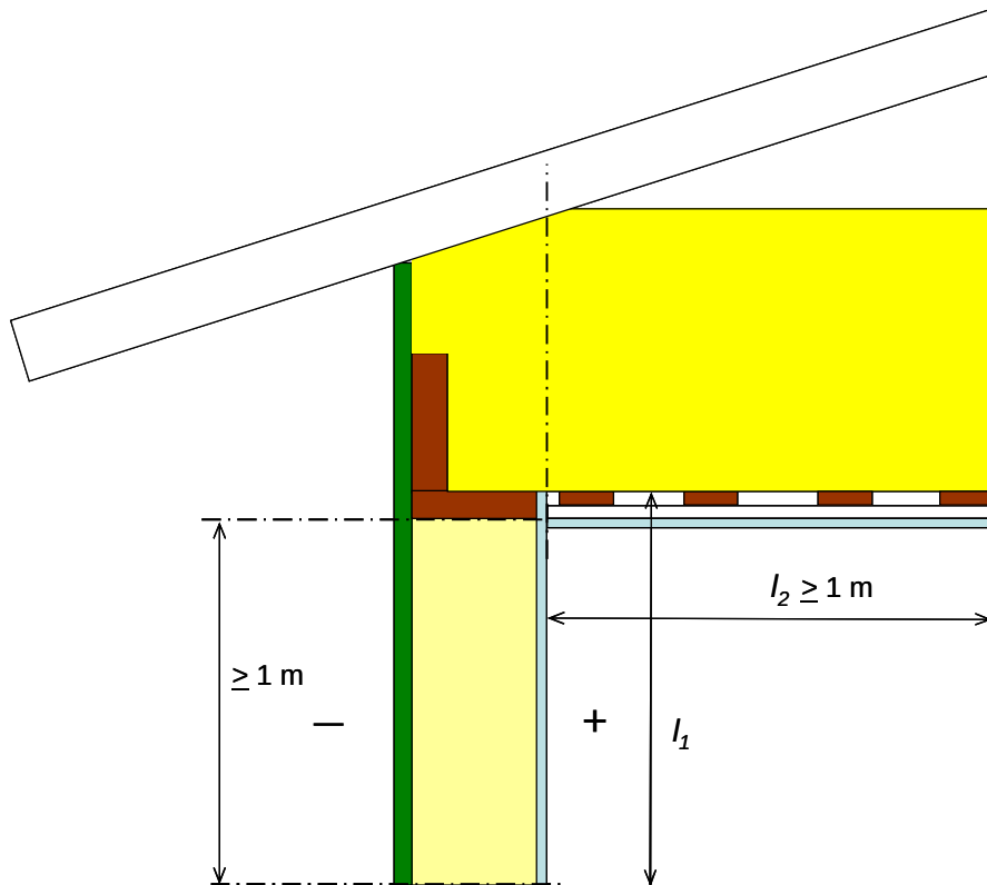
Kuva 7. Esimerkki ulkoseinän ja yläpohjan liitoksen kylmäsilasta. Seinän ja yläpohjan U-arvot lasketaan katkoviivojen välisen rakenteen perusteella. Vertailutilanteen lämpövirta lasketaan seinän ja yläpohjan U-arvojen ja mittojen l_1 ja l_2 mukaan.
