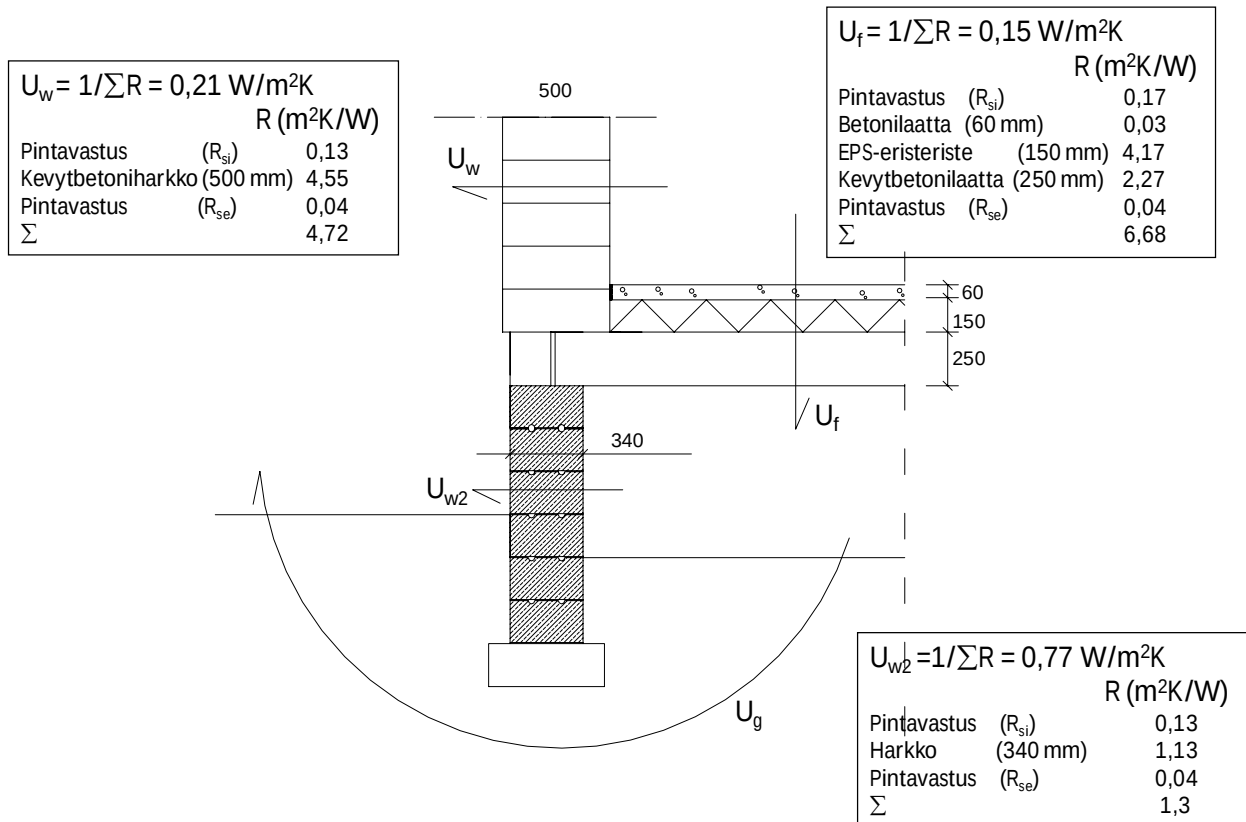
Kuva 73. Kevytbetonisen kiviseinän ja ryömintätilaisen alapohjan liittymä.
