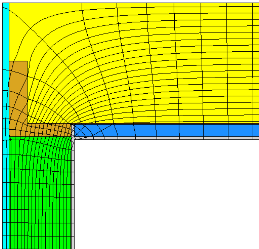
Kuva 26. Kuvan 24 tilanteen lämpötilojen tasa-arvokäyrät 1 asteen välein sekä niitä vastaan kohtisuorassa olevat lämpövirran virtaviivat. Kaikista virtaviivojen väleistä virtaa sama lämpövirta eli mitä tiheämmässä virtaviivat ovat sitä suurempi on lämpövirta. Ulkolämpötila on 0 °C ja sisälämpötila 20 °C.
