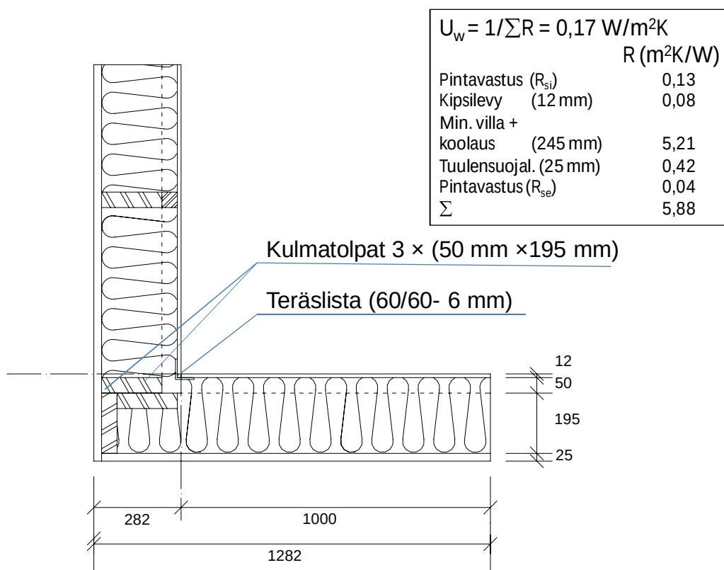
Kuva 20. Mallinnettava kahden puurankaisten ulkoseinän muodostama ulkokulma.
