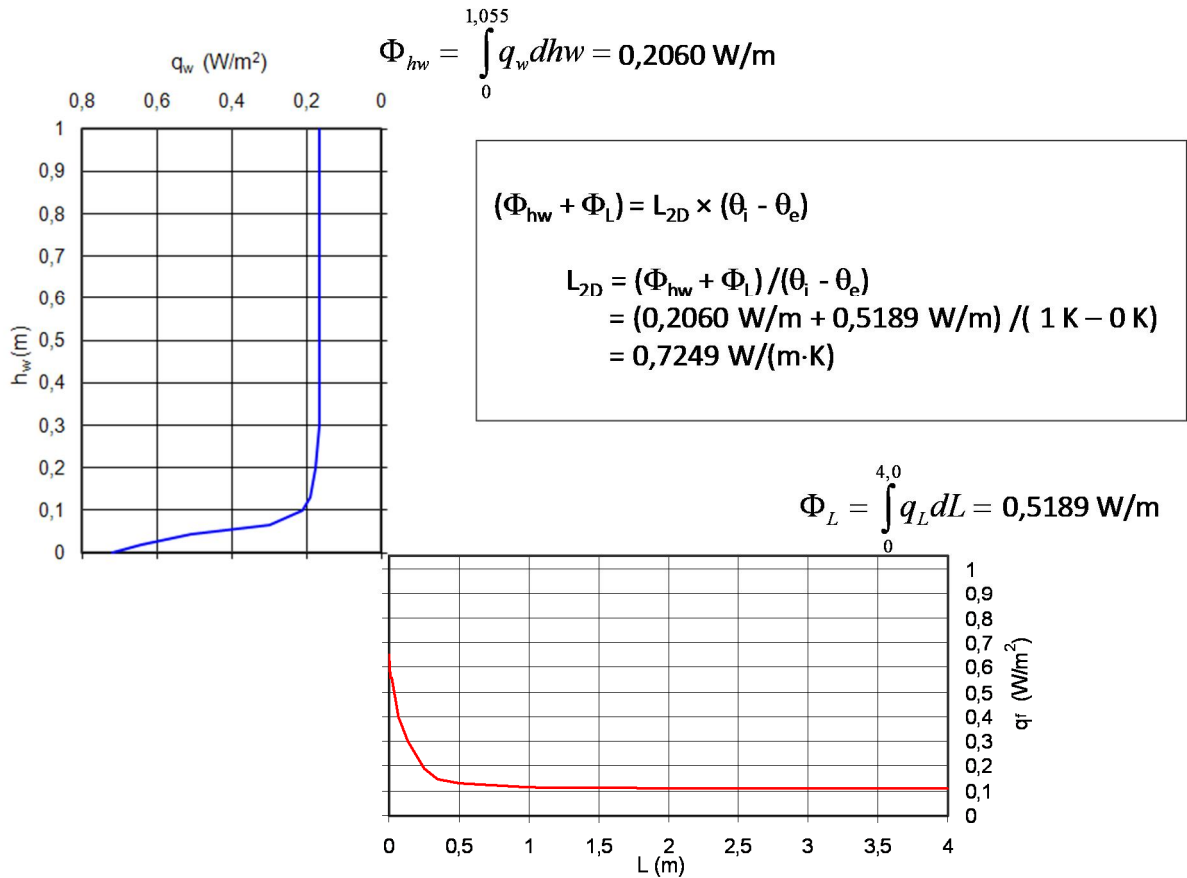
Kuva 16. Numeerisesti kaksikulotteisella elementtimenetelmällä määritetyt rakenteen sisäpintojen lämpövirtajakaumat ( q_f = lattiat ja q_w = seinä) ja rakenneosien yhteenlasketut lämpövirrat ( \Phi_{hw} ja \Phi_L ), sekä lämpöteknisen kytkentäkertoimen ( L_{2D} ) määrittäminen.
