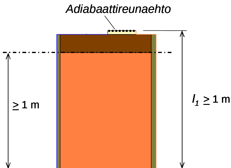
Kuva 10. Yksinkertaistettu menettely ikkunan liitoksen kylmäsillan laskentaan. Ikkuna korvataan adiabaattireunaehdolla ja karmen syvyytenä käytetään laskennallista karmisyvyyttä. Seinän U-arvo lasketaan pistekatkoviivojen välisen rakenteen perusteella. Vertailutilanteen lämpövirta lasketaan seinän mitan l_1 mukaan.
