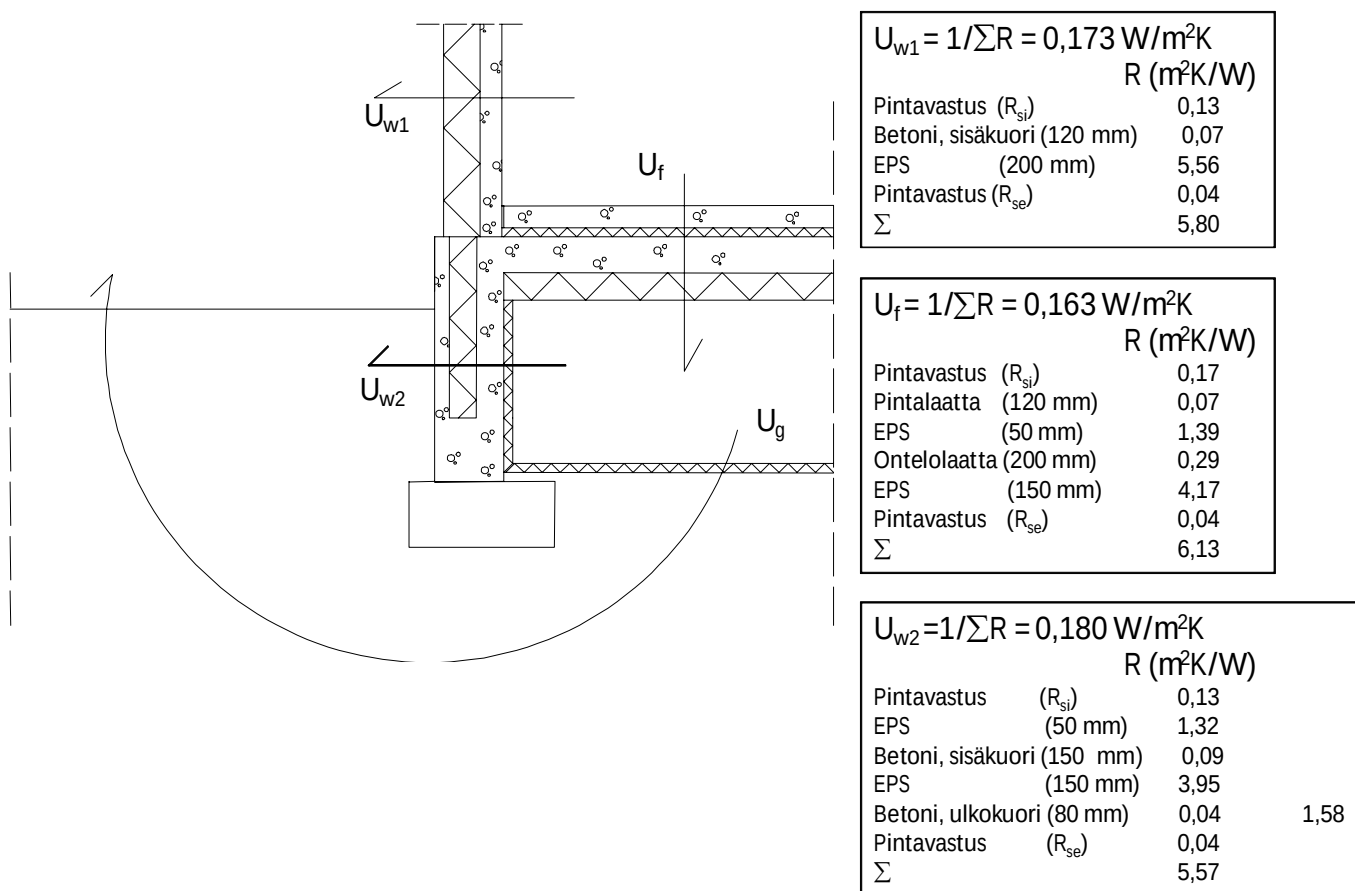
Kuva 43. Ryömintätilaisen alapohjan, eristetyin kiviseinän ja eristetyin pintalaatan liitos normaali-rakenteena.
