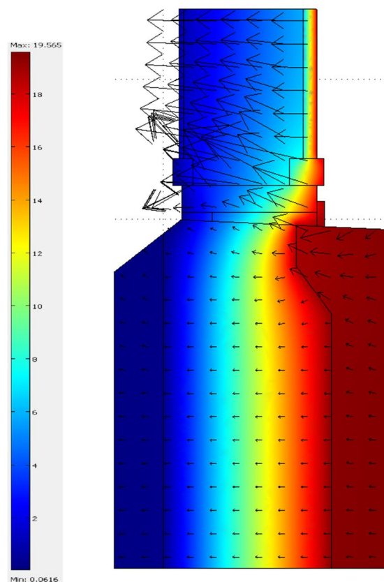
Kuva 58. Lämpötilat ja lämpövirtavektorit ilman karmikenkää taulukon 30 tilanteessa 2. Kaksiulotteinen laskenta.
