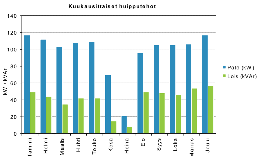
Kuva 8 Sähkön mitatut kuukausittaiset huipputehot ja loistehot.
