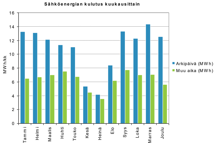
Kuva 7 Sähköenergian kulutus kuukausitasolla.
